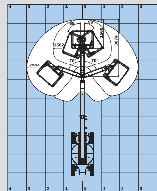
Opción 3D: Rotación pendular
